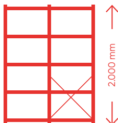
tot H = 2.000 mm: 1 Kruisschoor
