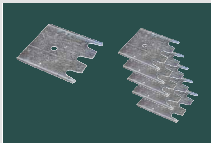
Onderlegplaten voor voetplaten voor het uitvullen van oneffenheden in de vloer + verzinkt
