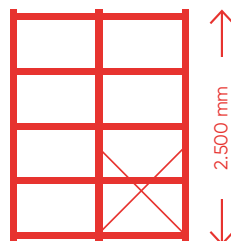
tot H = 2.500 mm: 1 Kruisschoor
