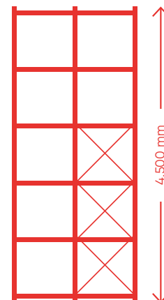
tot H = 4.500 mm: 3 Kruisschoren
