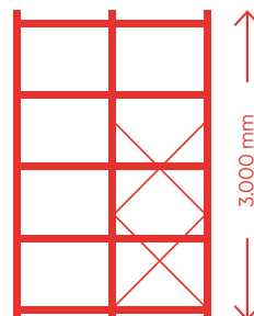
tot H = 3.000 mm 2 Kruisschoren
